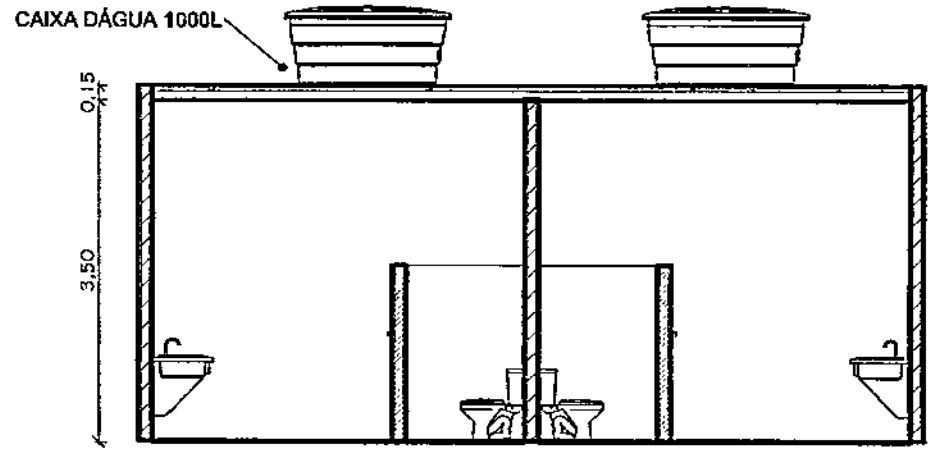
2 Corte AA 1 : 75
