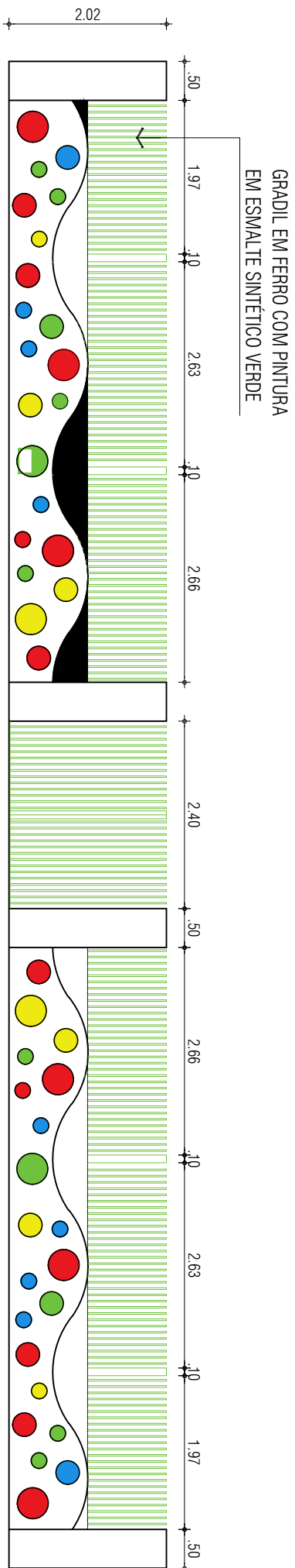
FACHADA LATERAL ATUAL
