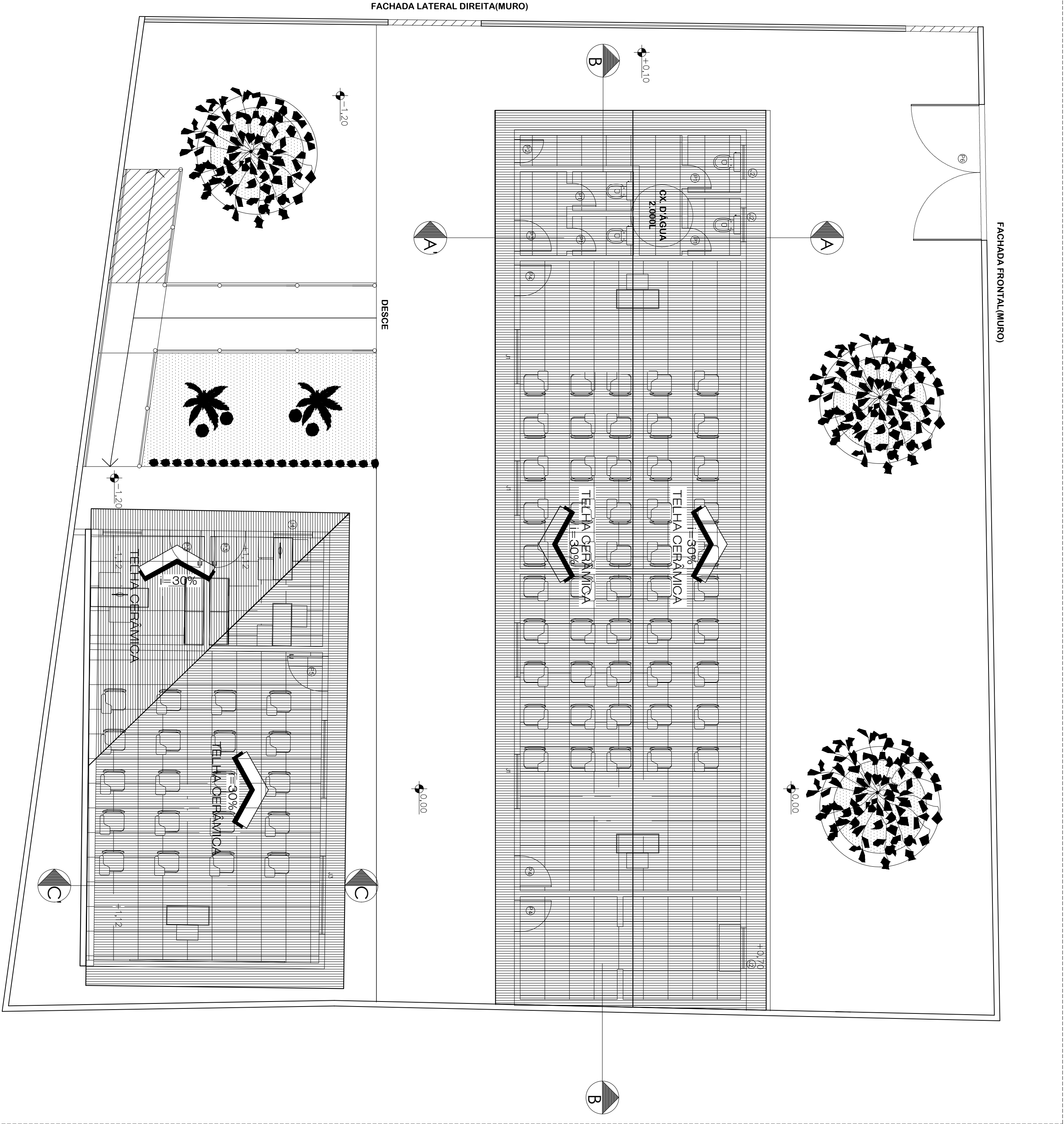
PLANTA DE COBERTURA
