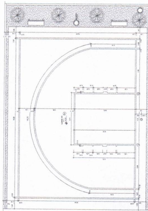
4 Planta Baixa - Quadra 3x3 Executivo
