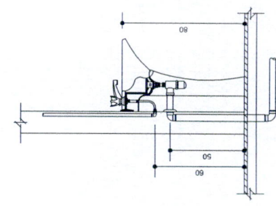
Detalhe Vaso Sanitário
